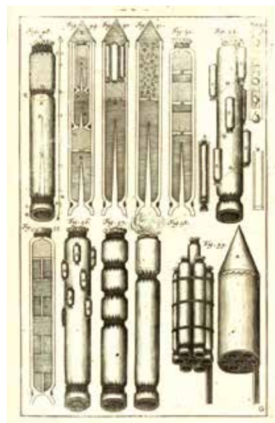
Рисунок из книги «Великое искусство артиллерии» К. Семеновича, показывающий устройство ракет
